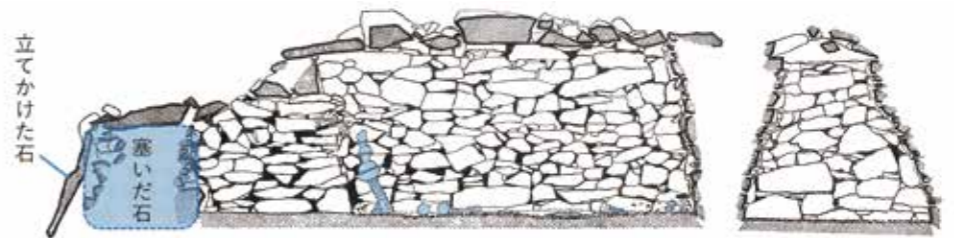
▲図2 中宮1号墳石室
